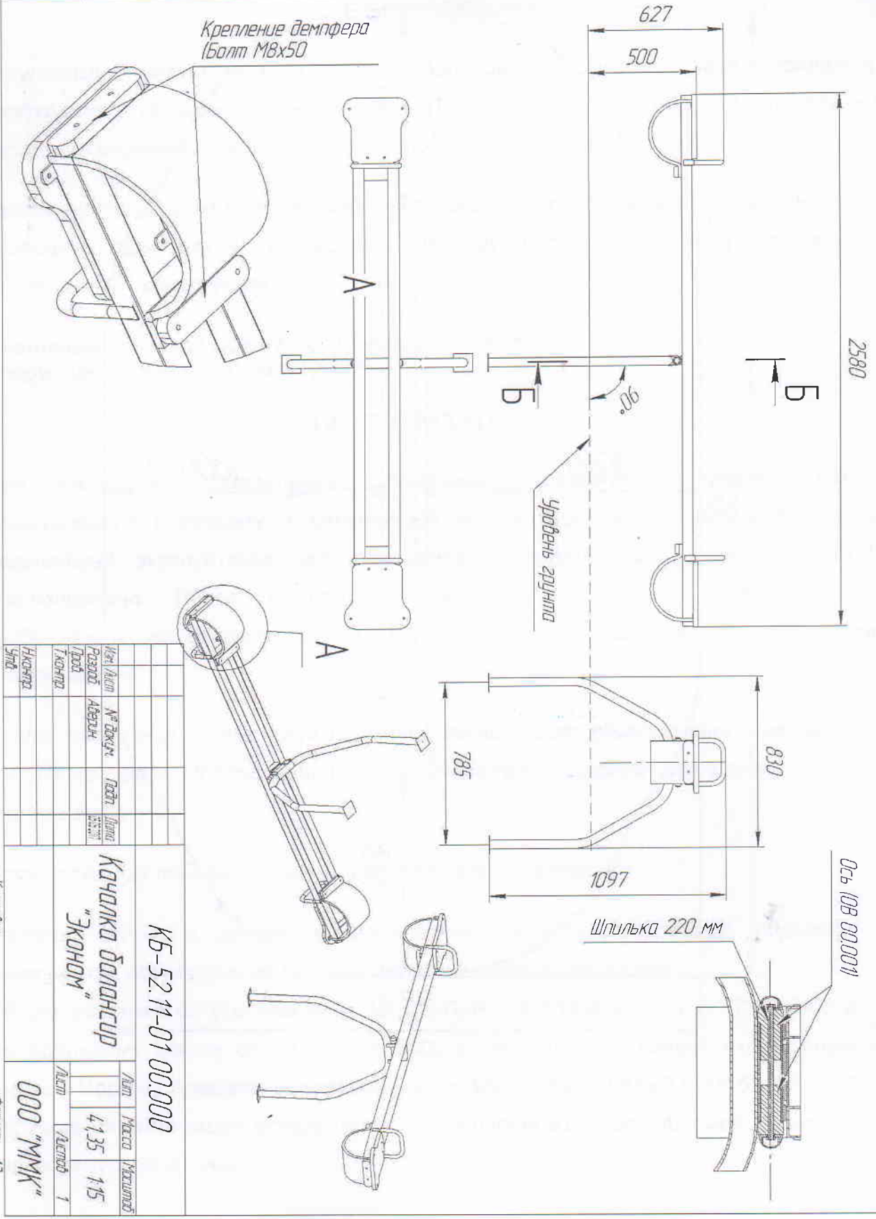
Рис №2 чертеж инструкции монтажа детской качалки-балансир
