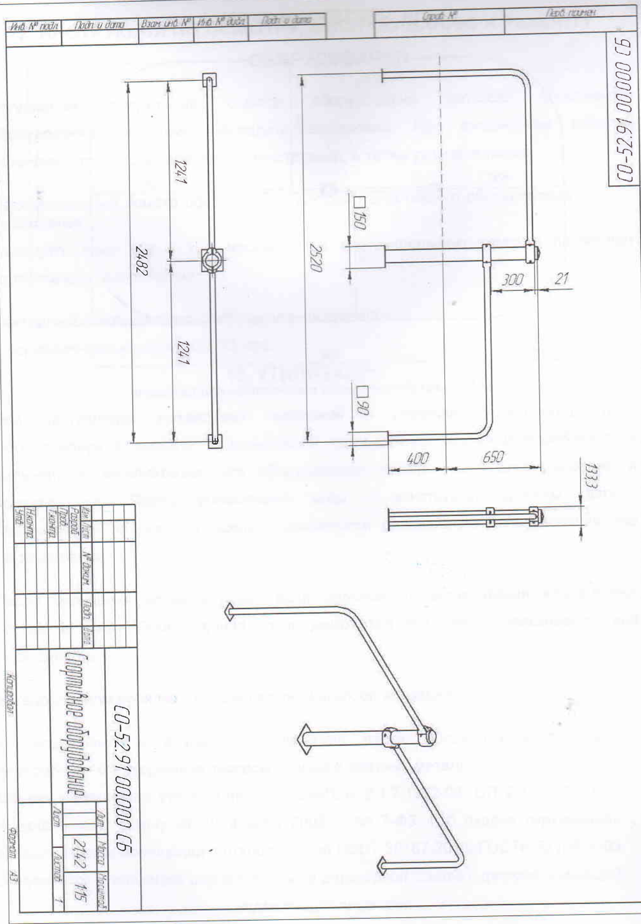
Рис №3 инструкция монтажа спортивного оборудования
