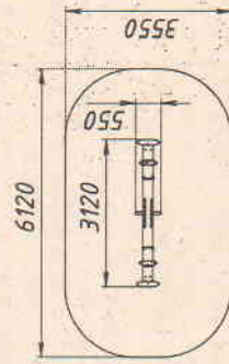
General view (Общий вид)
